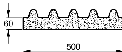
CORTE A - A'
